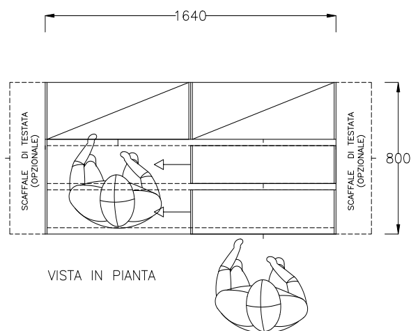
SCHEMA DIMENSIONALE
